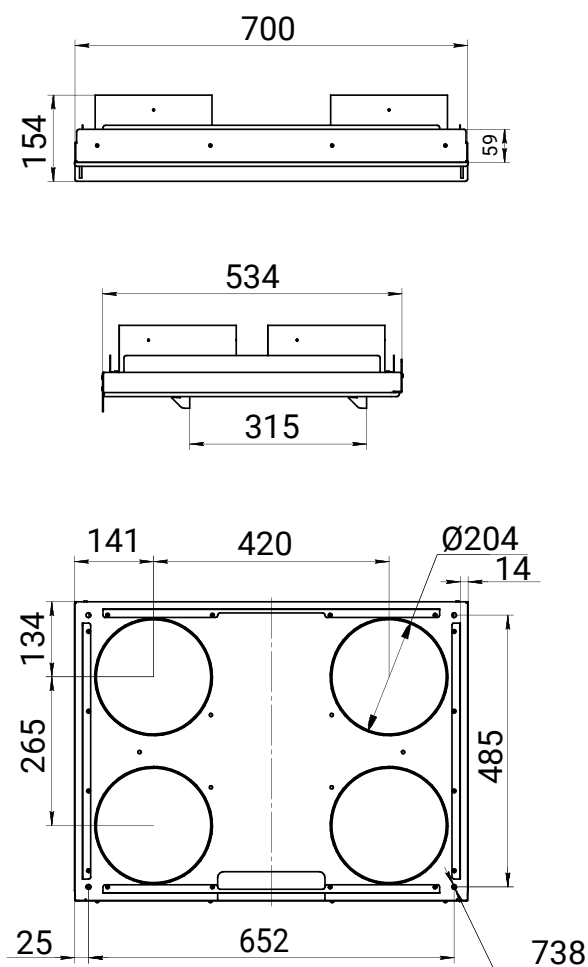
Монтажная панель ЕСТ МР-TOP 550:
