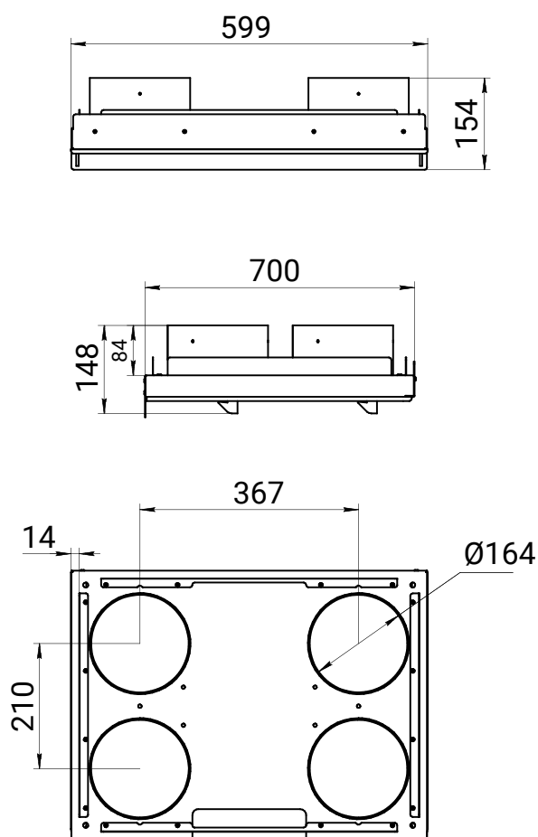
Монтажная панель ЕСТ МР-TOP 400:
